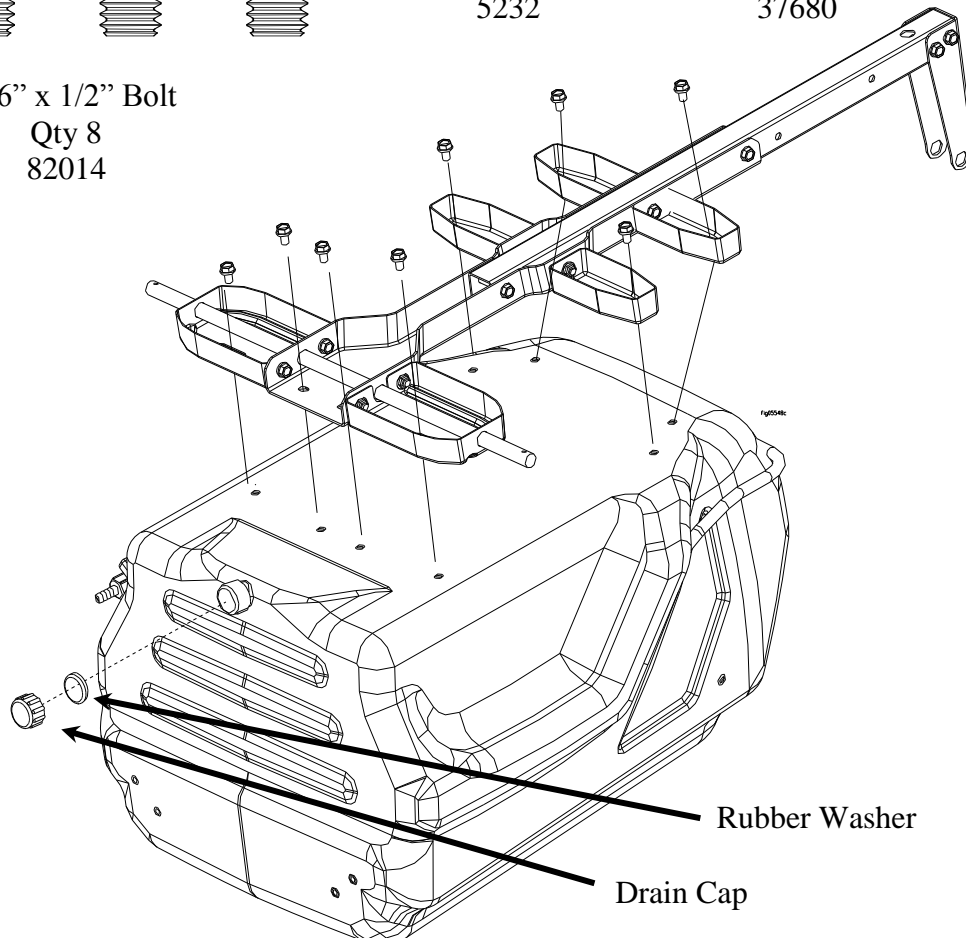
Rubber Washer Qty 5232
